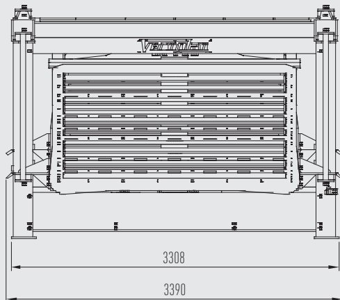
Frontansicht
