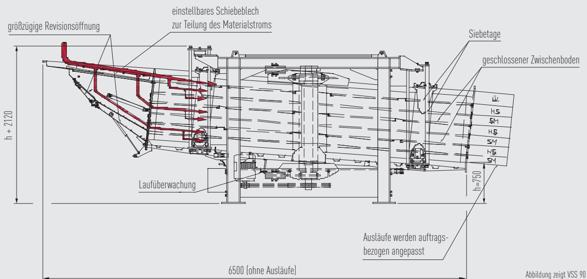
Seitenansicht
